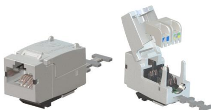
Connettore di tipo RJ45 Jack Keystone schermato
